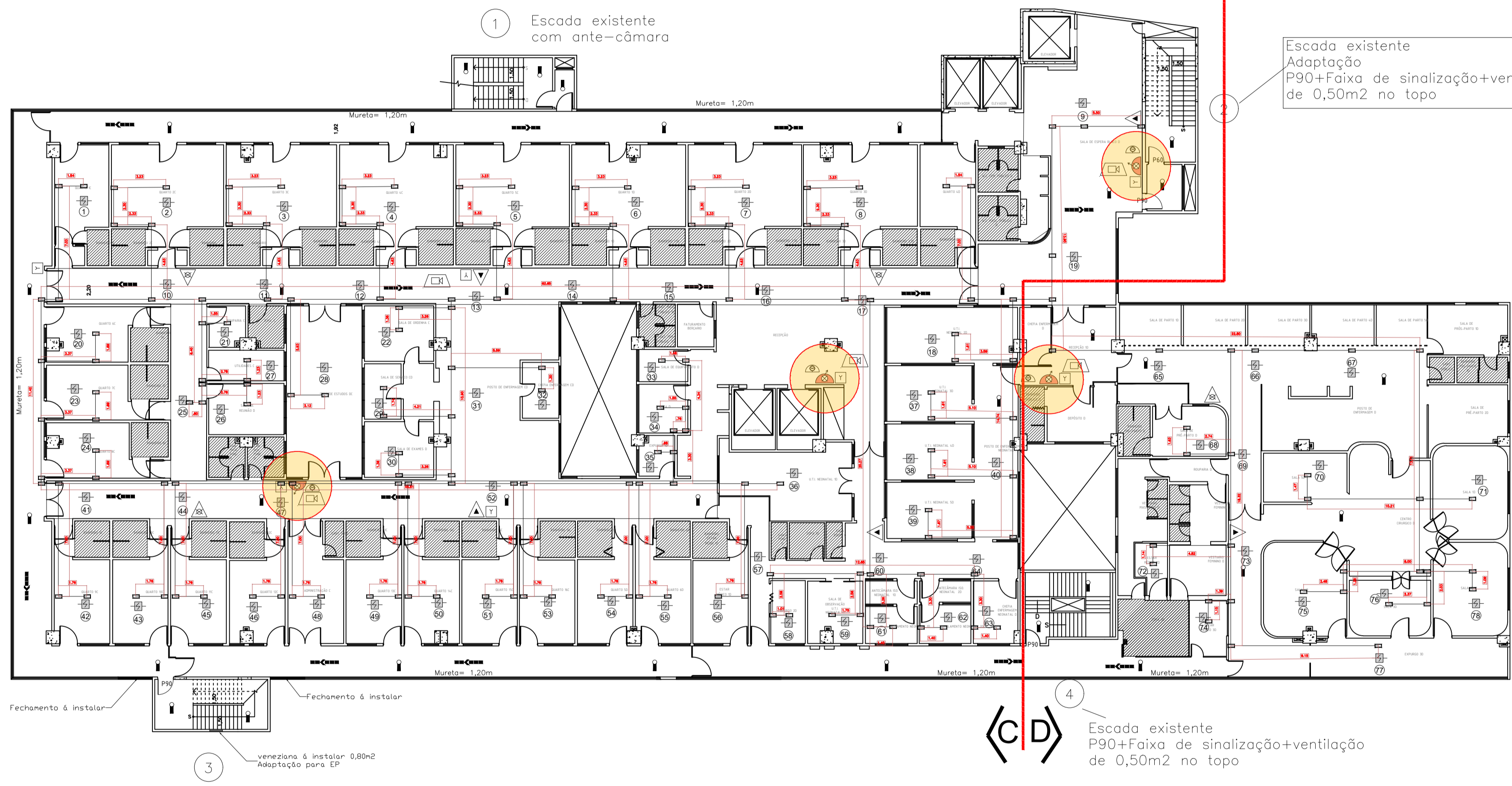
PLANTA LAYOUT - BLOCO CD - 6º PAVIMENTO ESCALA 1:200
